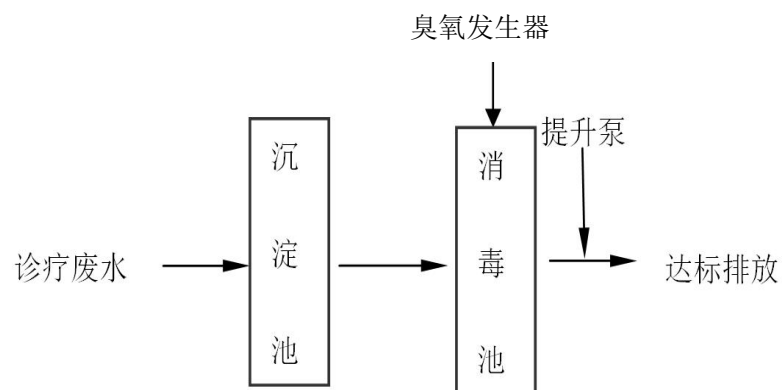
图4 项目污水处理工艺流程图
